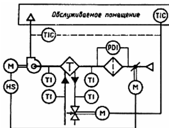
Пример выполнения принципиальной технологической схемы вентиляционной системы
